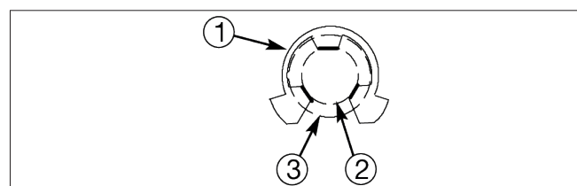
Fig. 11 Montage correct du clip
