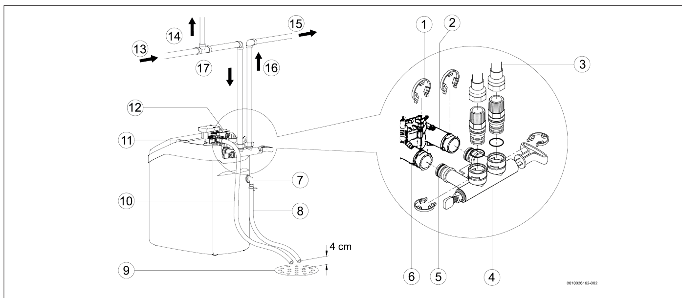
Fig. 7 Vue d'ensemble d'une installation standard
