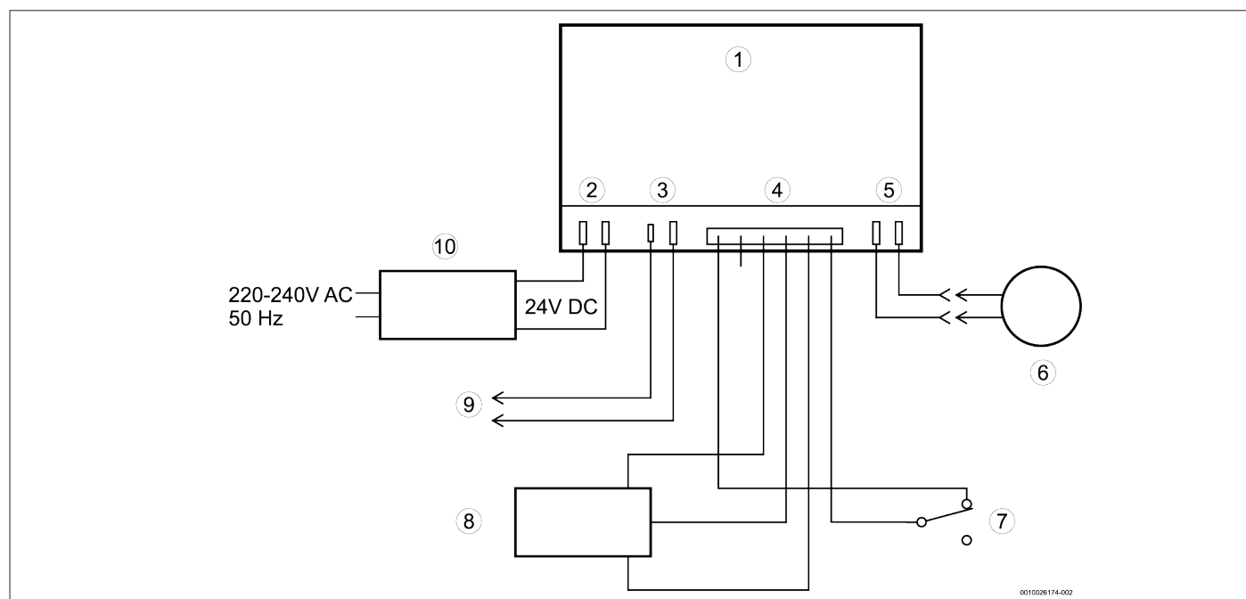
Fig. 47 Schéma de câblage
