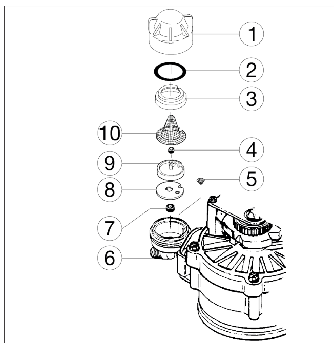
Fig. 39 Démontage de l'injecteur et du venturi
