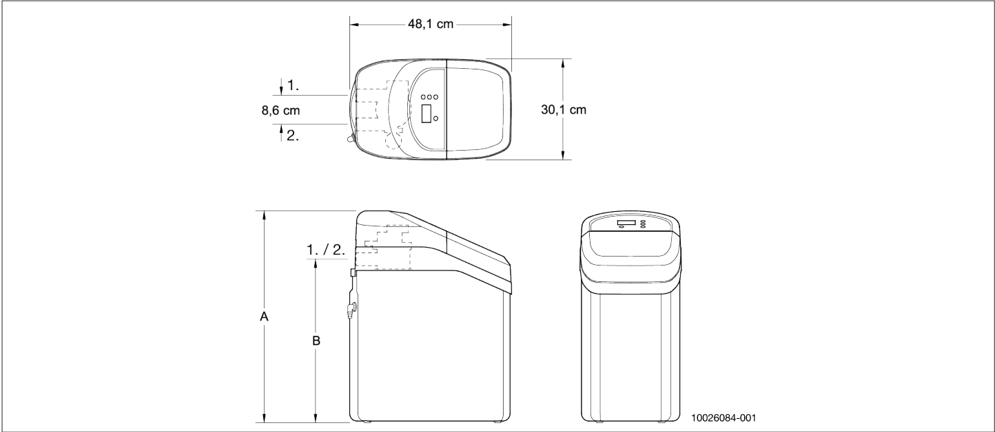
Fig. 1 Adoucisseur d'eau - vue de dessus, de côté et de face
